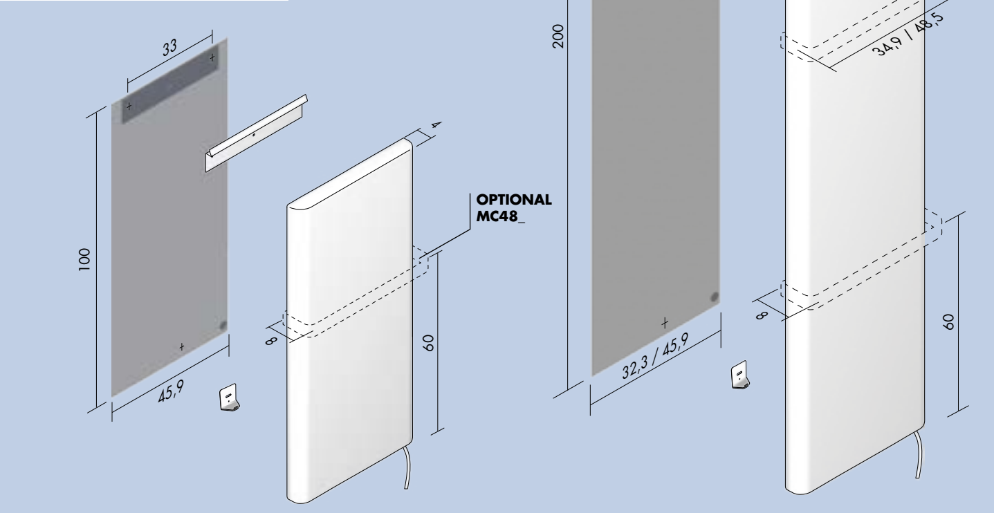
Electric with cable / Version électrique avec cable / Elektrische Ausführung mit Kabel / Versión electrica con cable
